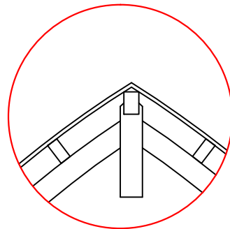
B SKALA 1:25
