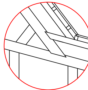
D SKALA 1:25
