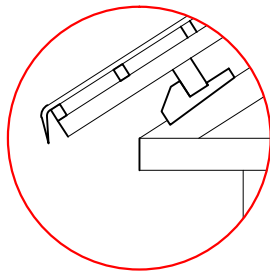
A SKALA 1:25
