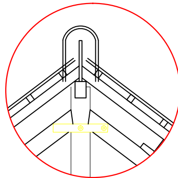
B SKALA 1:25
