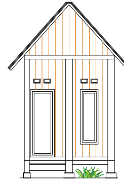
TAMPAK DEPAN SKALA 1:100
