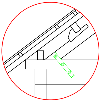
A SKALA 1:25
