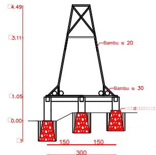
POTONGAN A-A SKALA 1:100
