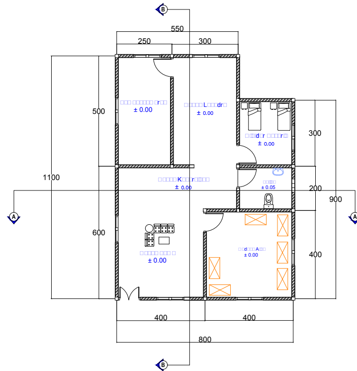
RUANG KEBERSIHAN SKALA 1:100
