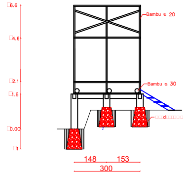
POTONGAN B-B SKALA 1:100
