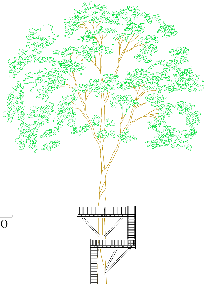
TAMPAK DEPAN FLYING FOX SKALA 1:200
