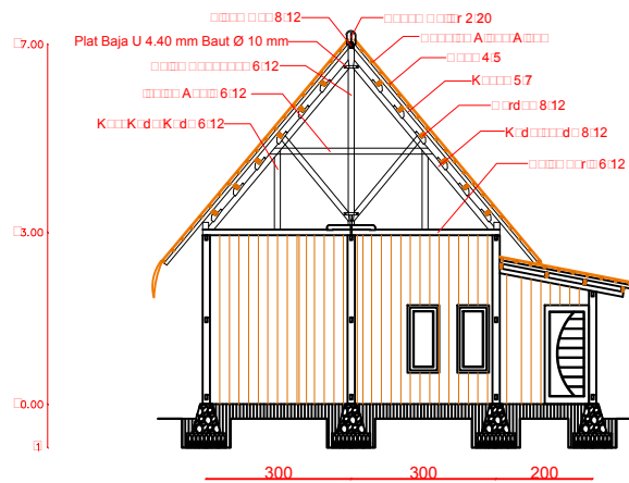
POTONGAN B-B SKALA 1:100
