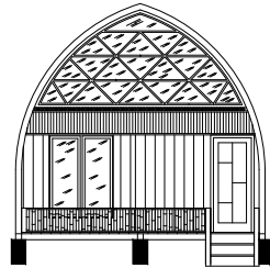
TAMPAK DEPAN SKALA 1:100
