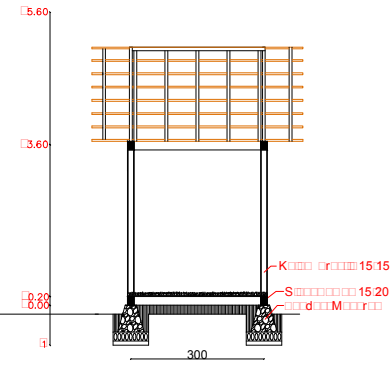
POTONGAN A-A
