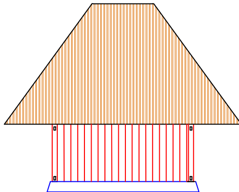
TAMPAK BELAKANG SKALA 1:100
